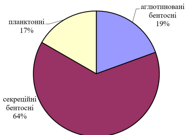
Комплекс форамініфер нижнього сantonу кар'єру смт Черкаське (останній уступ) (Донецька обл.). Зона Gavelinella infrasantonica
