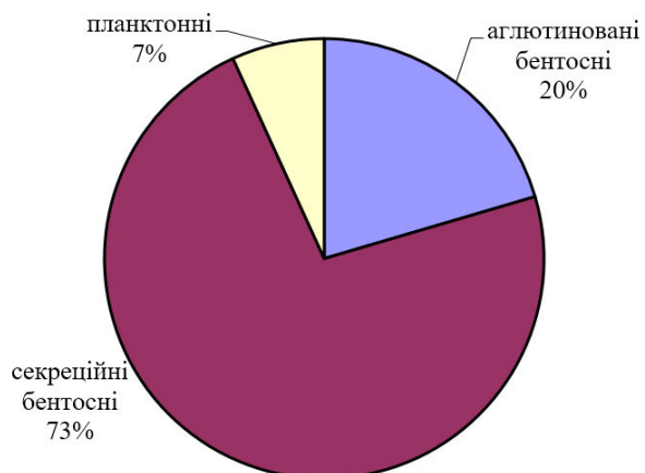
Комплекс форамініфер середнього кампану відслонення с. Збірне (Лутугинський р-н, Луганська обл.). Зона Brotzenella monterelensis
