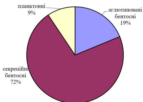
Комплекс форамініфер нижнього сantonу Білогорівський кар'єр Лисичанського содового заводу с. Білогорівка (Луганська обл.). Зона Gavelinella infrasantonica
