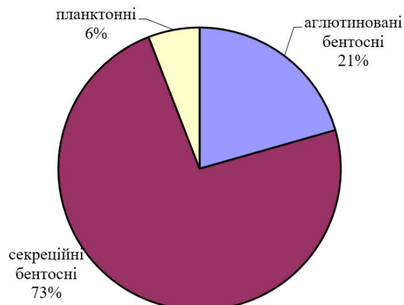
Комплекс форамініфер верхнього кампану кар'єру поблизу смт Георгіївка (Лутугинський р-н, Луганська обл.). Зона Globorotalites emdyensis
