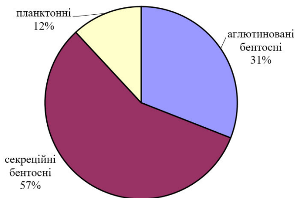
Комплекс форамініфер середнього кампану відслонення с. Збірне (Лутугинський р-н, Луганська обл.). Зона Brotzenella monterelensis
