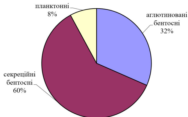
Комплекс форамініфер нижнього кампану кар'єру Балаклійського цементно-шиферного комбінату (Харківська обл.), зр. 8–10. Зона Cibicidoides temirensis
