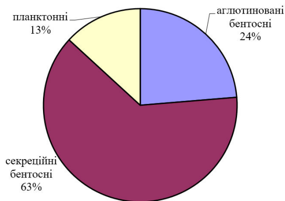
Комплекс форамініфер середнього кампану відслонення с. Сидорове (Слов'янський р-н, Донецька обл.). Зона Brotzenella monterelensis
