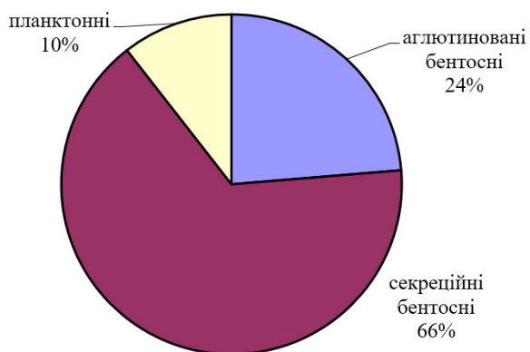
Комплекс форамініфер нижнього сantonтону кар'єру с. Мілова (Харківська обл.). Зона Gavelinella infrasantonica
