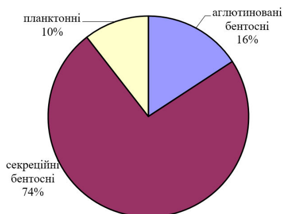
Комплекс форамініфер нижнього маастрихту свердловина 22-Д м. Суходільськ (Луганська обл.), зр. 04552 (гл. 88,4 м). Зона Neoflabellina reticulata
