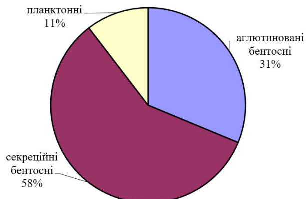
Комплекс форамініфер нижнього маастрихту свердловина 22-Д м. Суходільськ (Луганська обл.), зр. 04552 (гл. 88,4 м). Зона Neoflabellina reticulata
