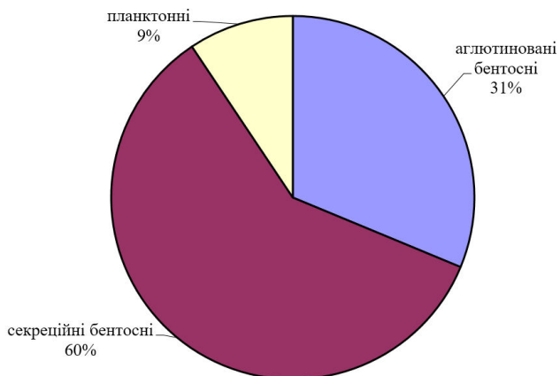
Комплекс форамініфер нижнього сantonу кар'єру смт Черкаське (останній уступ) (Донецька обл.). Зона Gavelinella infrasantonica
