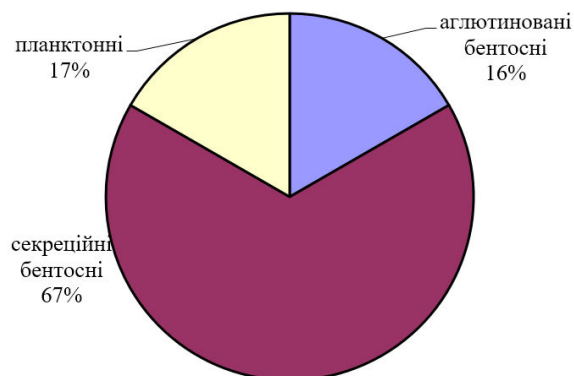
Комплекс форамініфер нижнього маастрихту зведеного розрізу відслонень с. Шандриголове (Краснолиманський р-н, Донецька обл.), зр. 9. Зона Brotzenella complanata
