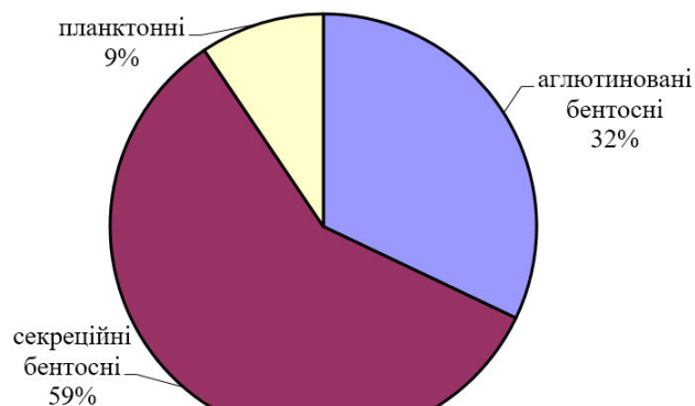
Комплекс форамініфер нижнього маастрихту відслонення Кам'яний брід (околиці м. Луганськ). Зона Brotzenella complanata
