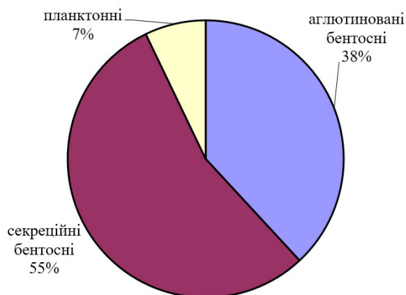
Комплекс форамініфер нижнього маастрихту зведеного розрізу відслонень с. Шандриголове (Краснолиманський р-н, Донецька обл.), зр. 6, 7, 8. Зона Neoflabellina reticulata
