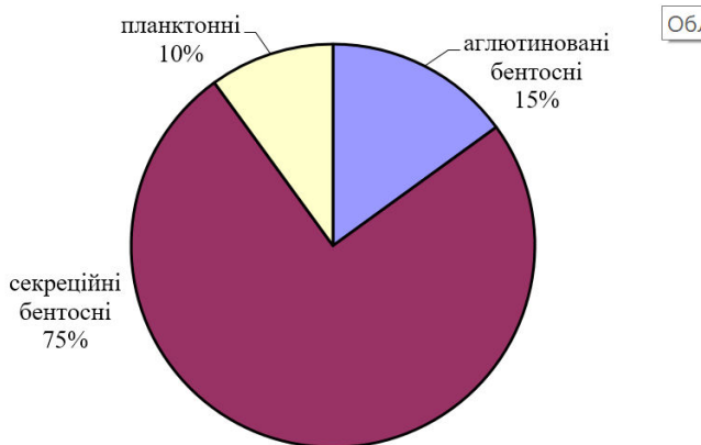
Комплекс форамініфер нижнього кампану відслонення с. Маяки (Донецька обл.). Зона Cibicidoides temirensis
