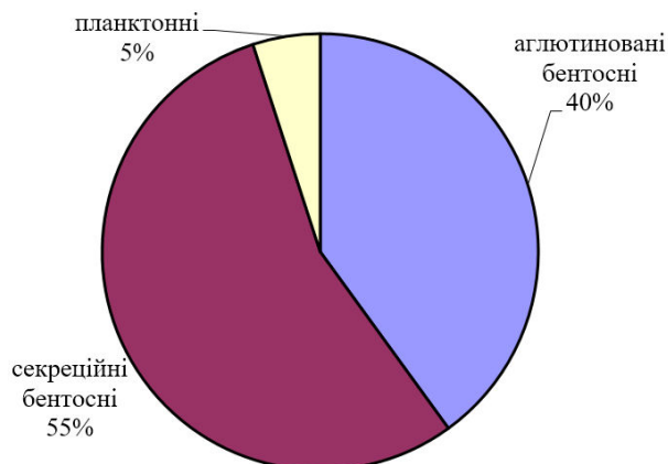
Комплекс форамініфер нижнього маастрихту зведеного розрізу відслонень с. Шандриголове (Краснолиманський р-н, Донецька обл.), зр. 6, 7, 8. Зона Neoflabellina reticulata
