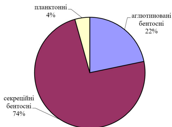
Комплекс форамініфер верхнього сantonу (нижня частина) кар'єру Балаклійського цементно- шиферного комбінату (Харківська обл.) зр. 2,3, 4-6. Зона Gavelinella stelligera
