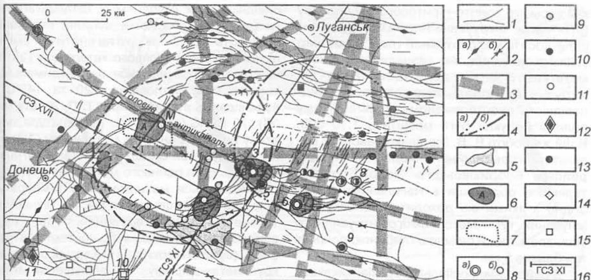
Рис. 1. Структурна схема домезозойської поверхні центральної частини ДСО з елементами мінерагенії 1 – диз'юнктивні порушення різних кінематичних типів за даними геологічного картування; 2 – осі пліквативних структур: а) антиклінальних, б) синклінальних; 3 – глибинні розломи за геофізичними даними; 4 – кільцеві структури регіонального рангу: а) Шахтарська, б) Нагольчанська; 5 – ділянки поширення дайок Міуського лампрофірового комплексу; 6 – приховані інтрузивні тіла в товщі осадових порід; 7 – ділянка аномально високого палеотеплового потоку за даними В. О. Привалова та ін. [12]; 8 – а) родовища, б) рудопрояви; ендегенна мінералізація: 9 – золото (родовища: 4 – Гостробугорське, 6 – Бобрівське; М – Михайлівський рудопрояр); 10 – свинець і цинк (родовища: 3 – Єсаулівське, 7 – Нагольчанське, 9 – Барило-Крепінське); 11 – срібло; 12 – уран (родовище: 11 – Миколаївське); 13 – ртуть (родовища: 1 – Костянтинівське, 2 – Микитівське рудне поле); 14 – сурма; 15 – фтор (родовище: 10 – Покрово-Кирейівське); 16 – лінії розрізів
