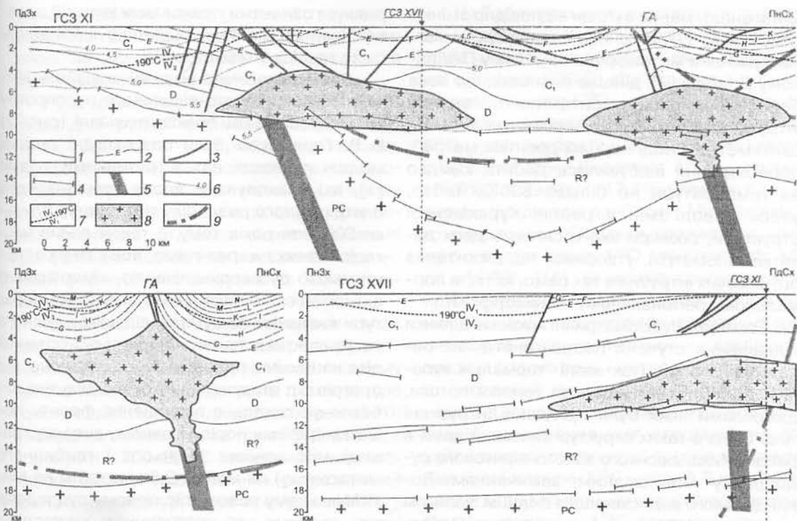
Рис. 2. Геологічні розрізи по лініях профілів ГСЗ XI, XVII та по лінії I-I
